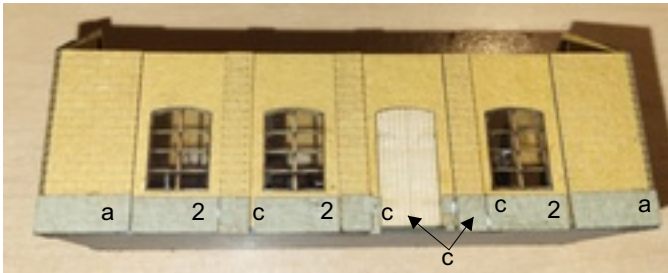
7. Sockel seitlich aufkleben. 1 a und c auf die Verkleidungen. Teile 2 unter die Fenster. Glue the base to the side. 1 a and c on the panels. Part 2 under the windows
