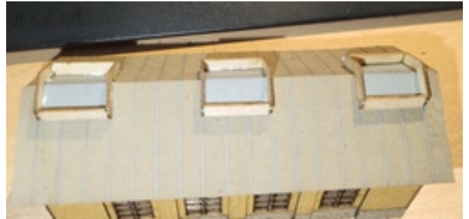
11. Die Dachhutzen aufkleben. Glue on the roof scoops.
